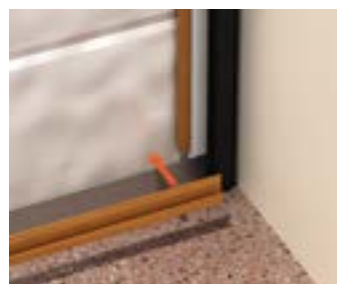
Устанавливаем нижний профиль для облицовки в стык с нижним профилем ворот, соблюдая технологический зазор в 1 мм до боковой крышки с каждой стороны
