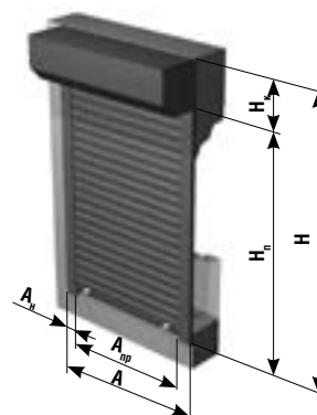
Накладной монтаж
